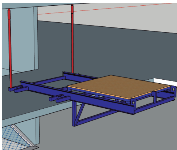
INSTALACIÓN EN LOSA
