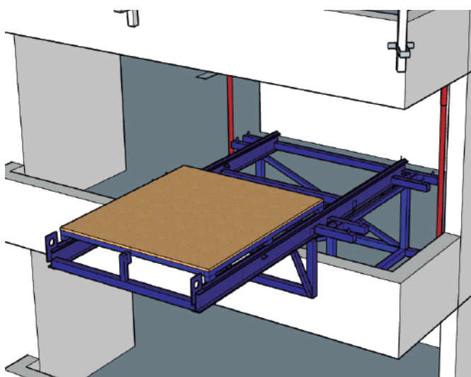
INSTALACIÓN EN ANTEPECHO
